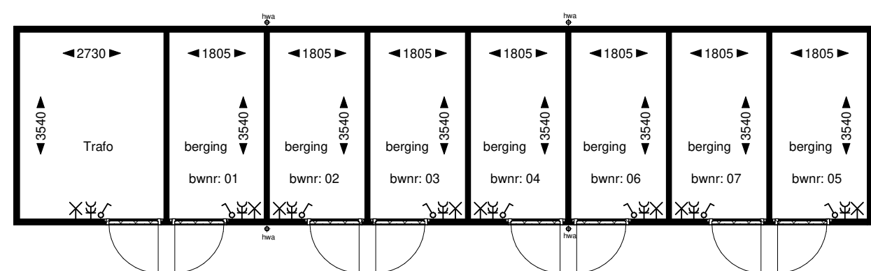
Begane grond
