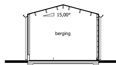
Doorsnede A-A
