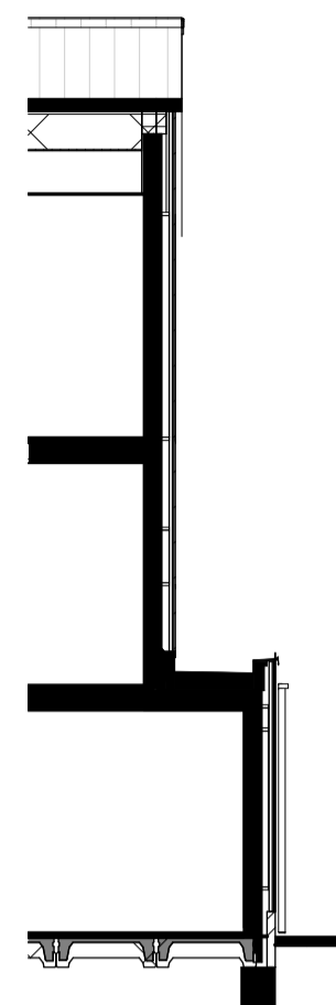
Doorsnede
