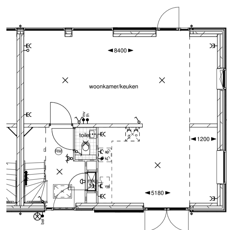
Begane grond
