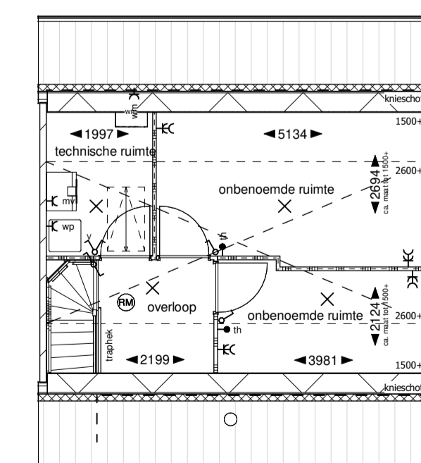
Tweede verdieping bnr 5 gesp. en 8
