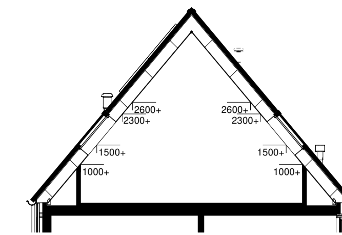
Doorsnede
