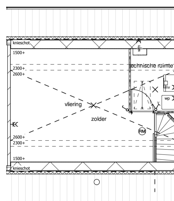
Tweede verdieping
