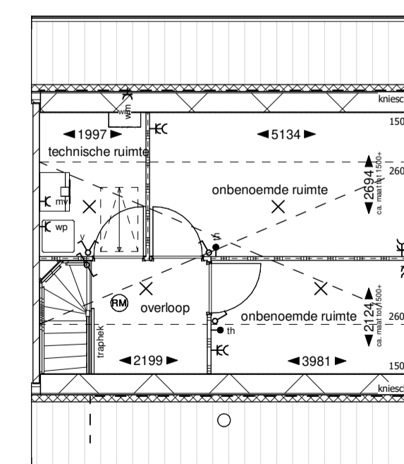
Tweede verdieping bnr 6 en 7 gesp.
