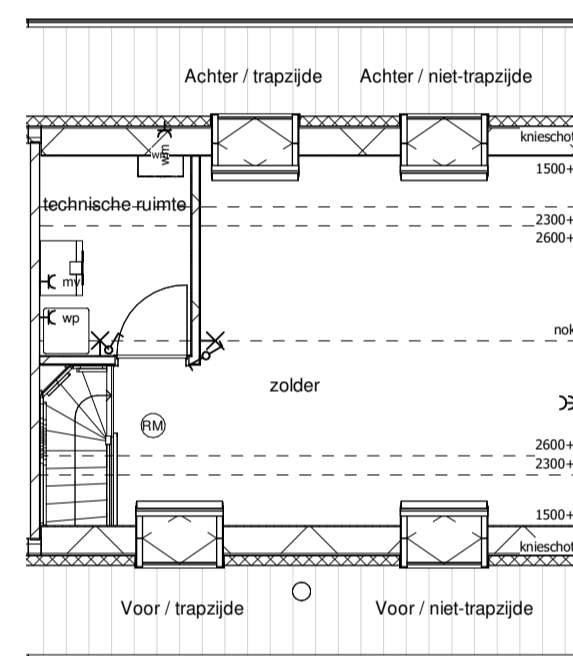
Tweede verdieping
