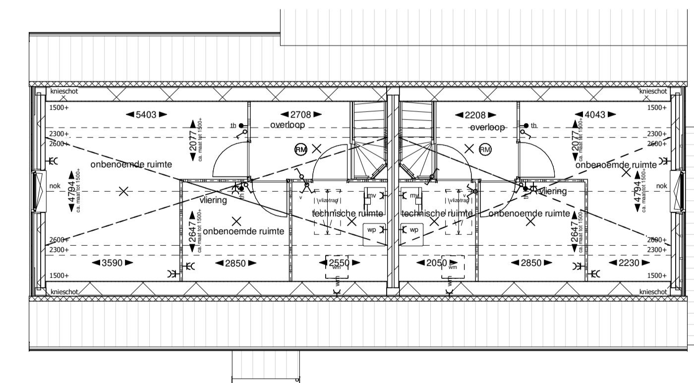
Tweede verdieping
