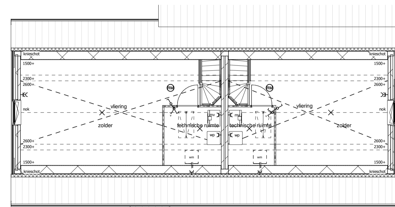
Tweede verdieping
