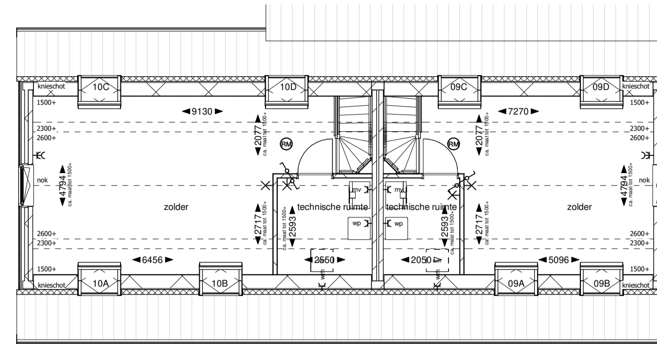
Tweede verdieping
