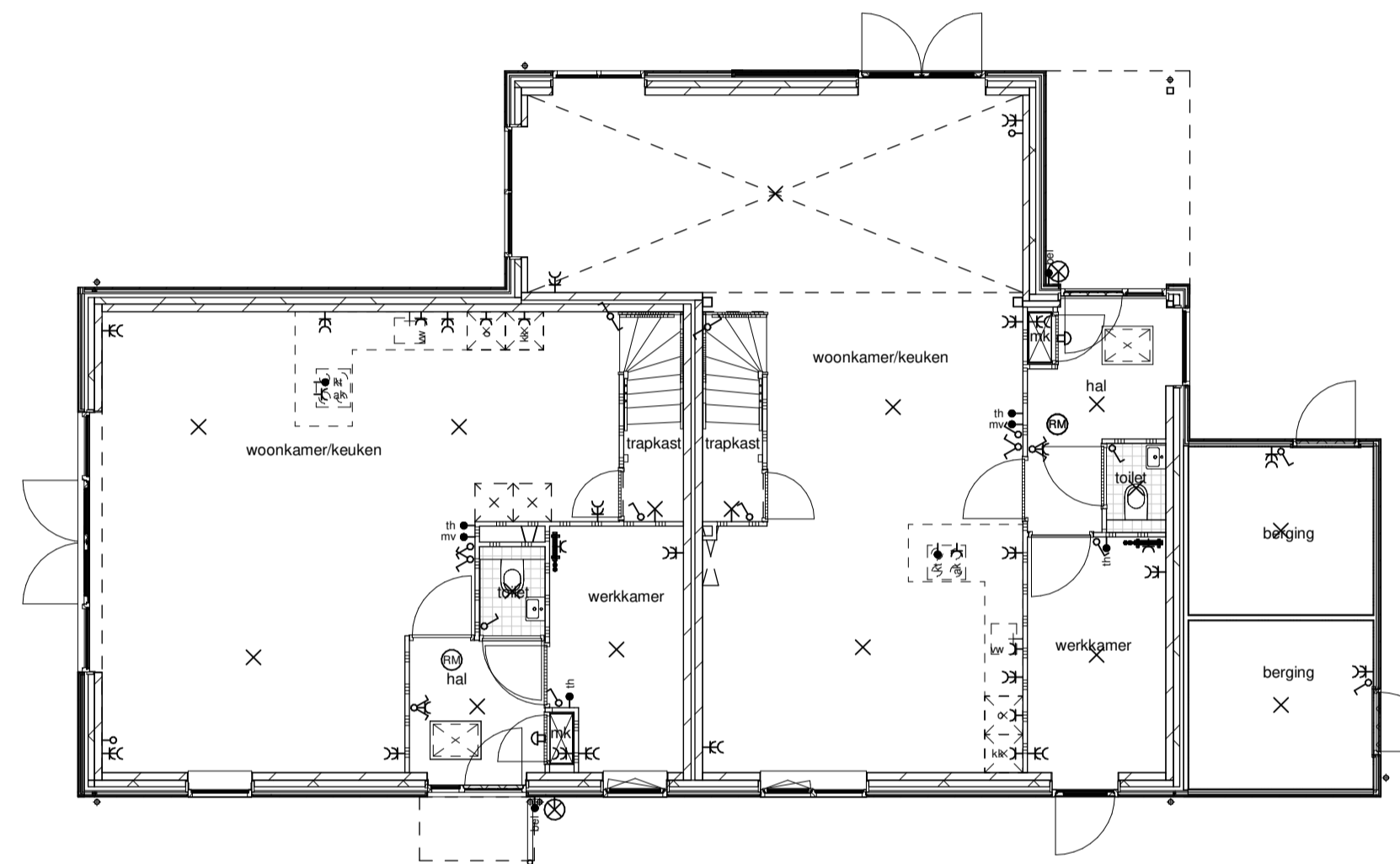
Begane grond
