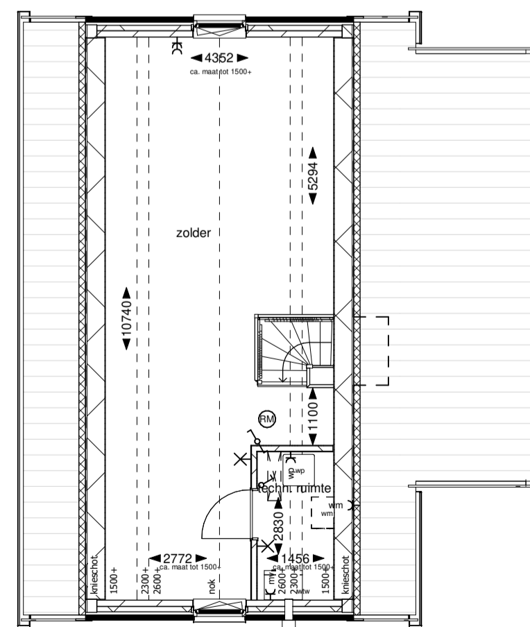
Tweede verdieping
