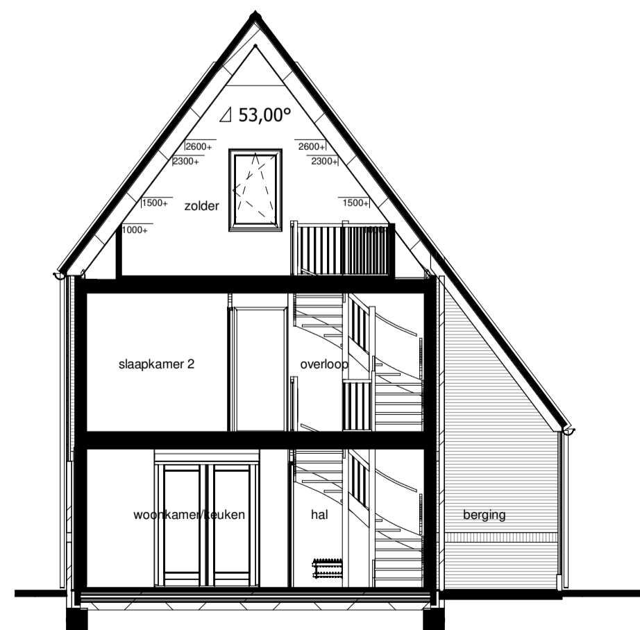
Doorsnede B-B
