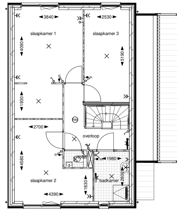
Eerste verdieping
