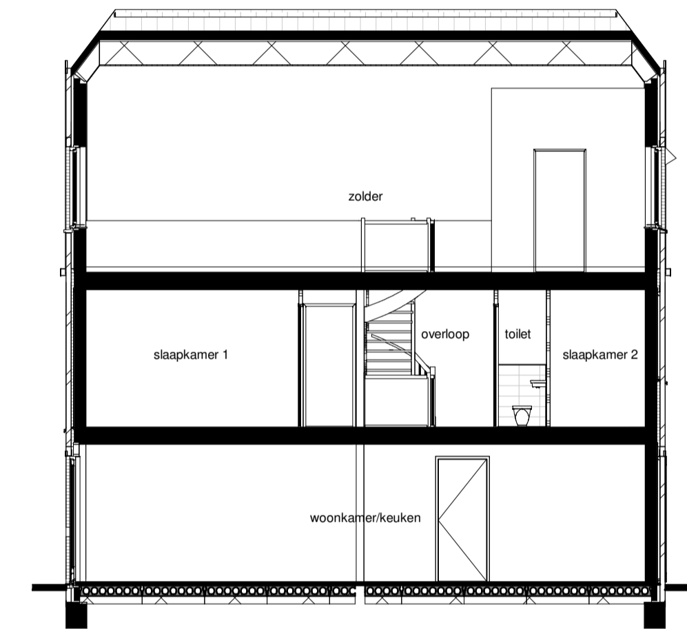
Doorsnede A-A
