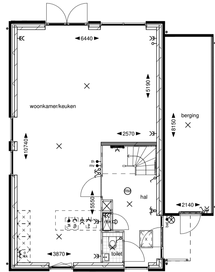
Begane grond
