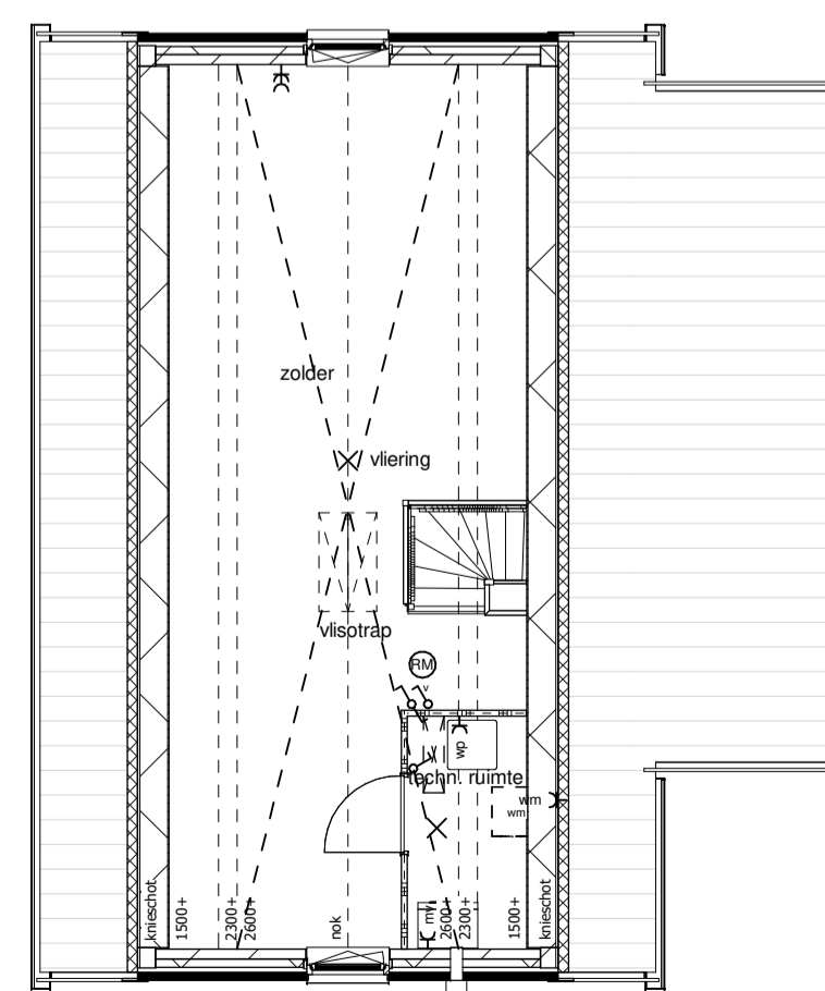
Tweede verdieping
