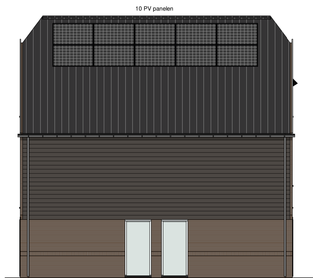
Linker zijgevel
