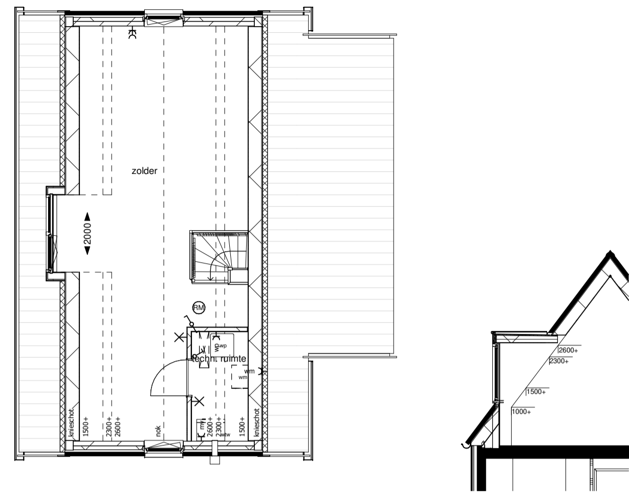
Tweede verdieping
