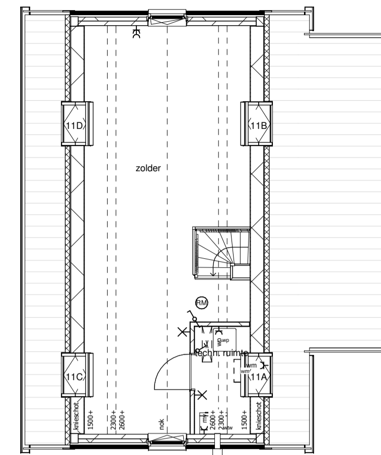
Tweede verdieping
