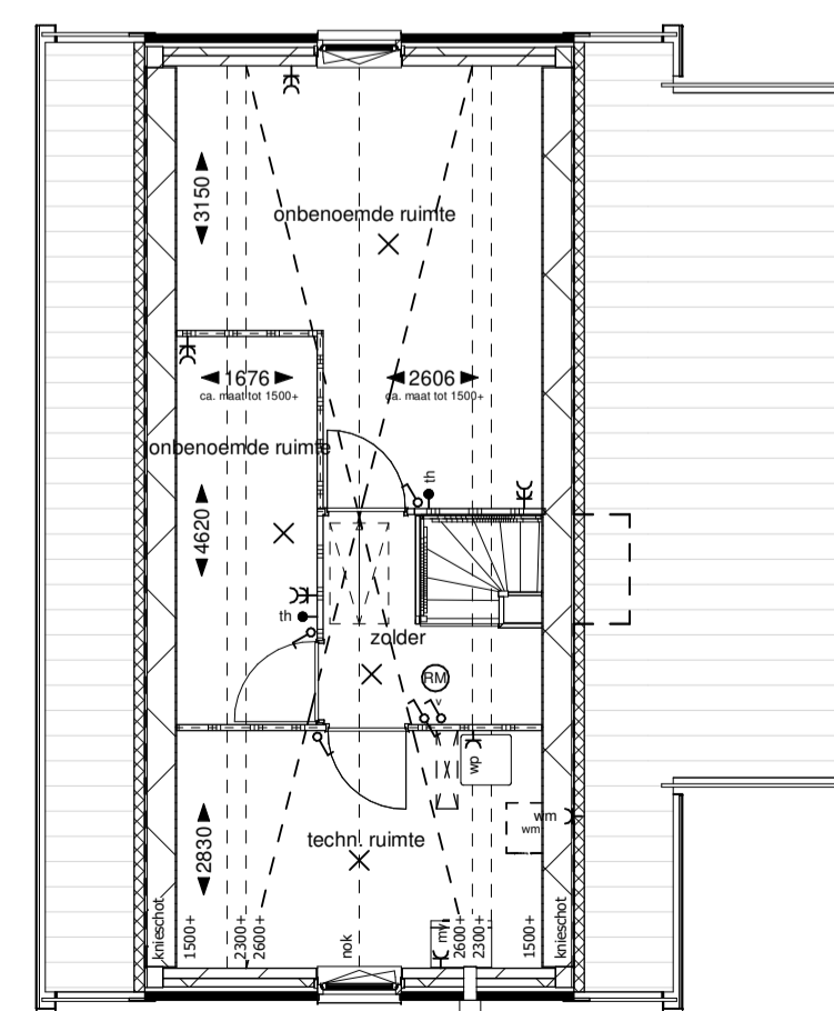
Tweede verdieping
