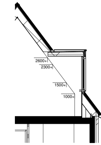
Doorsnede DE
