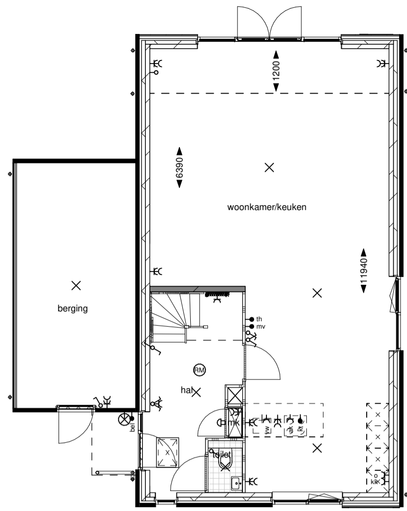
Begane grond
