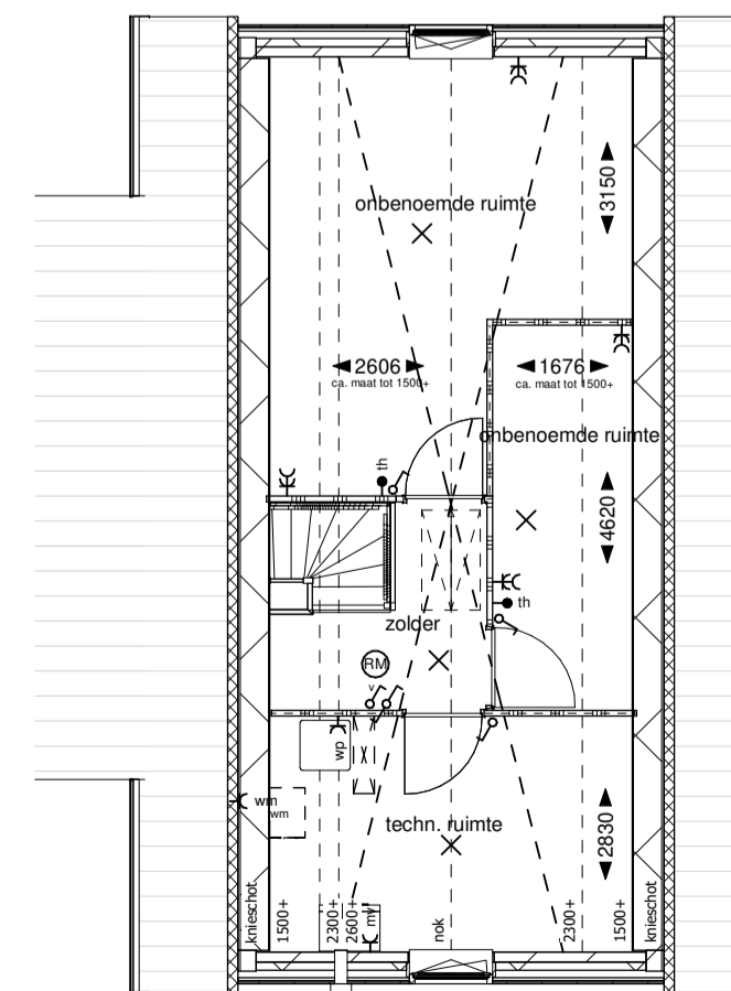
Tweede verdieping
