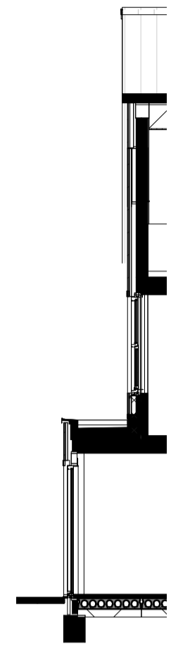
Doorsnede E
